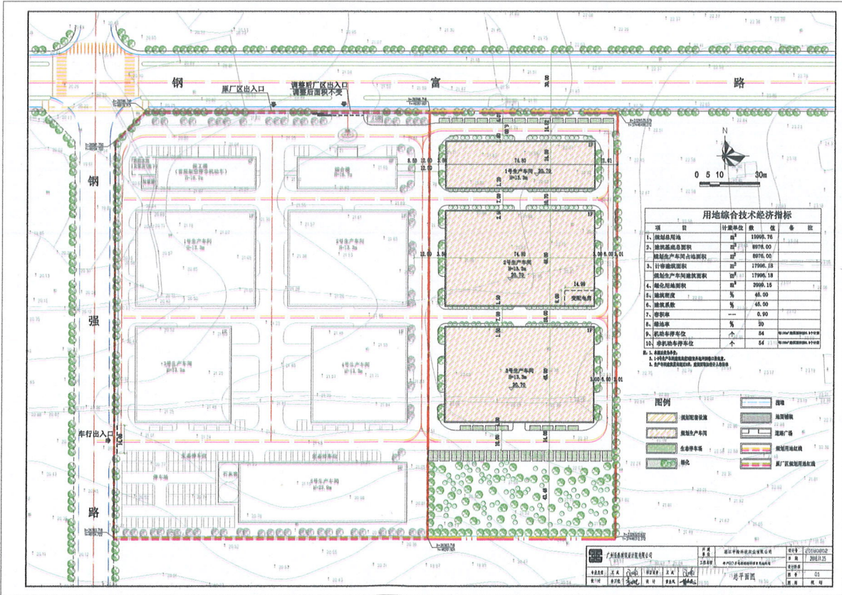
总平面图
