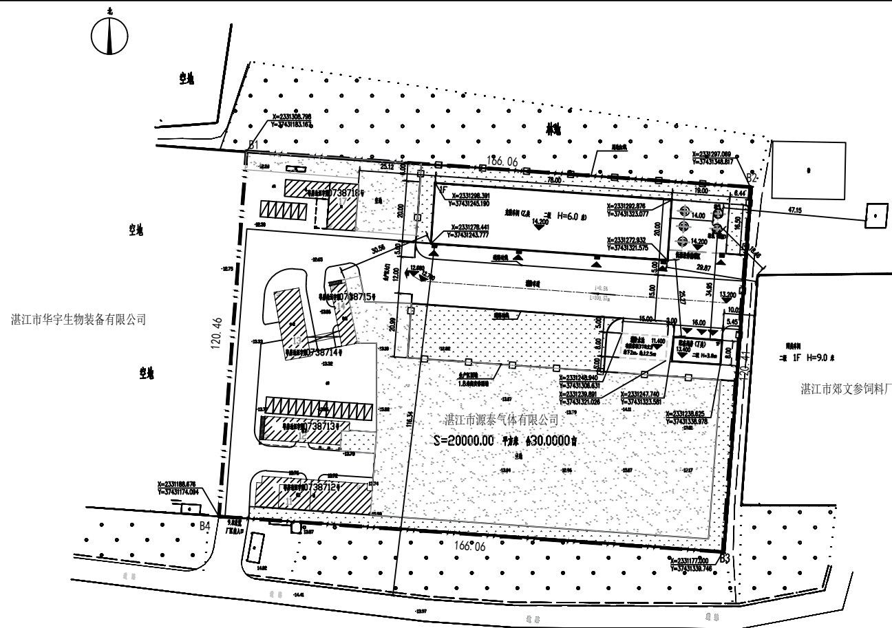
湛江市源泰气体有限公司东海岛工业气体充装站临时建筑规划总平面图和效果图
