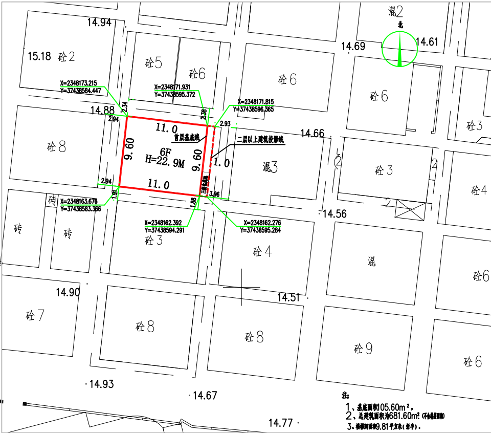
总平面图
