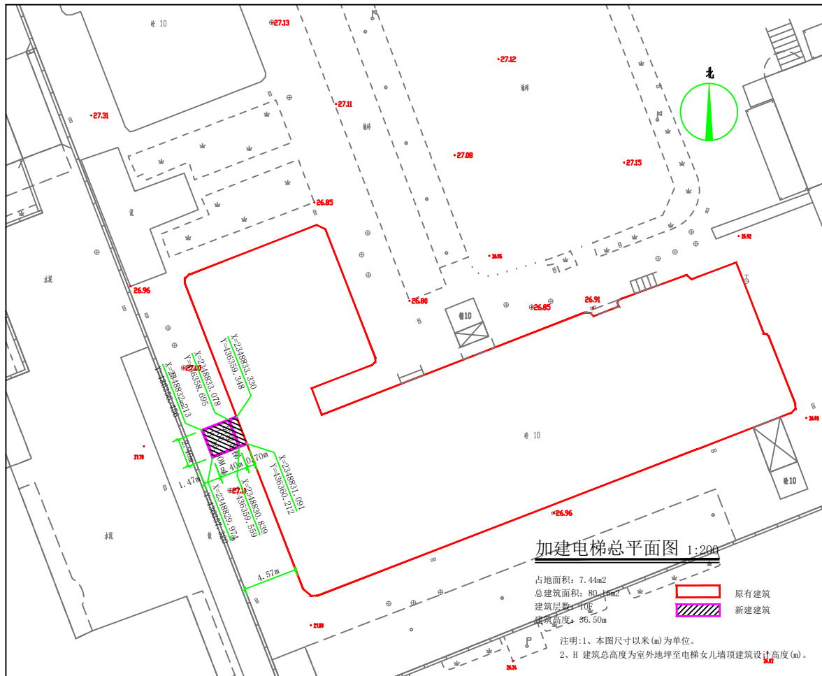
总平面图
